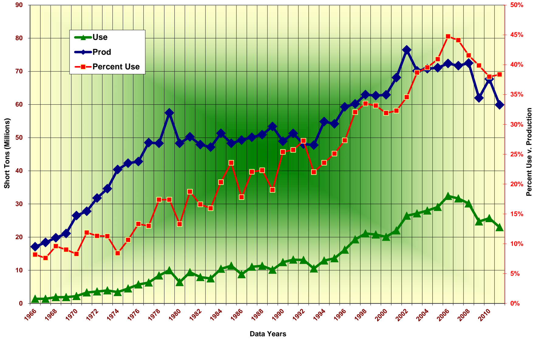
ACAA Fly Ash Production & Use Comparisons 1966-2011
